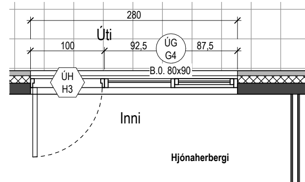
G4 H3 Plan 1 : 50
