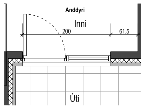
ÚH H1 Plan 1 : 50
