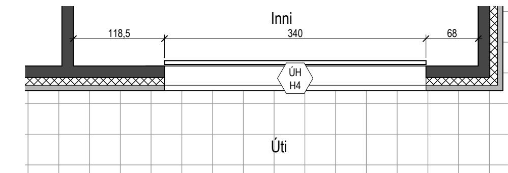
ÚH- H4 Plan 1 : 50
