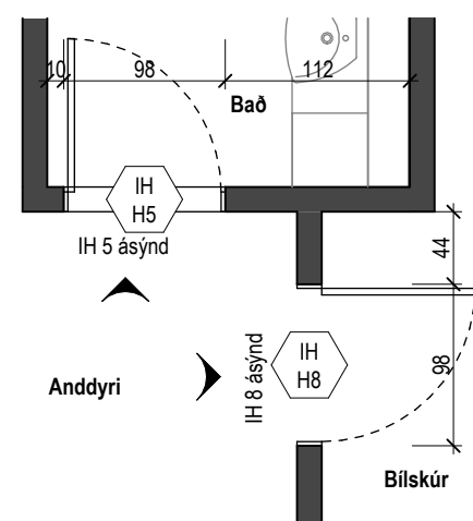
IH H5 og H8 - Plan 1 : 50
