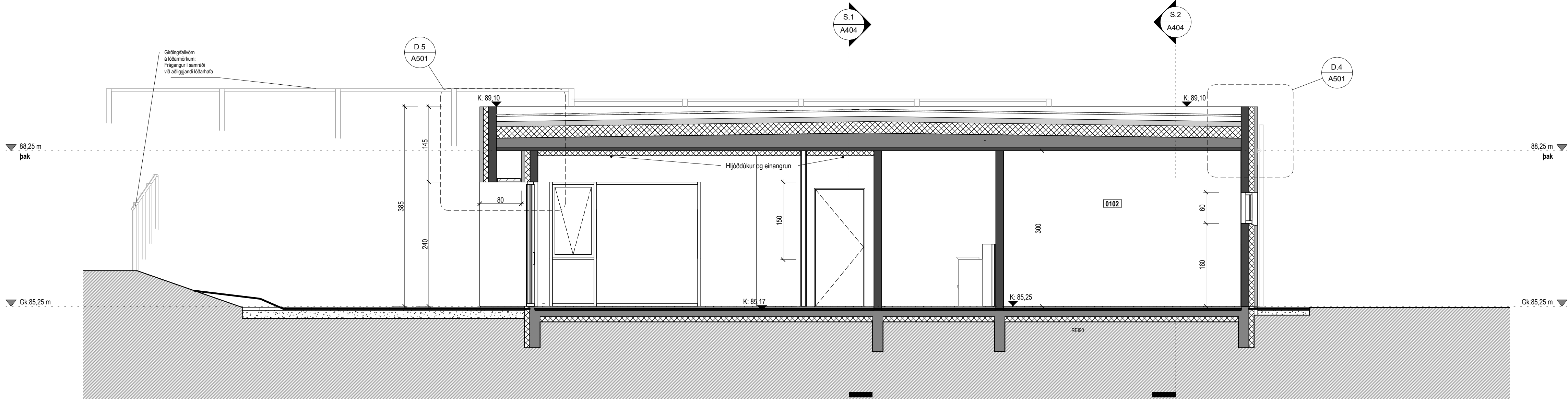
Snið 3 1 : 50
